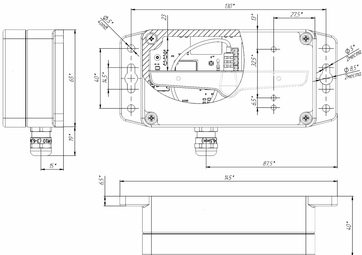
Рисунок 2 — Чертеж общего вида РМИ NB-IoT
