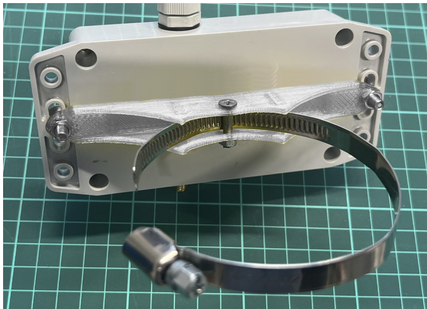
Рисунок 3 — Кронштейн для универсального монтажа
