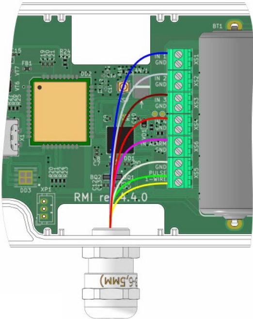
Рисунок 5 — Подключение проводов к клеммам модуля РМИ NB-IoT
